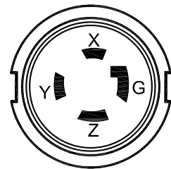
NEMA L15-30P PSE
