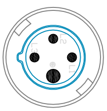
IEC60309 60A
