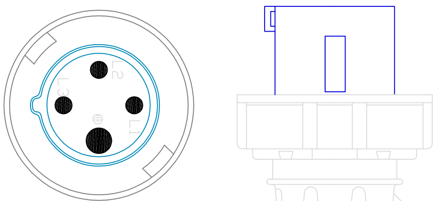
IEC60309 60A
