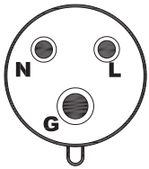
IEC60309 16A
