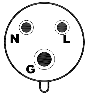
IEC60309 16A
