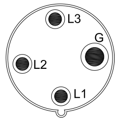
IEC60309 60A 3P (2)
