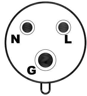
IEC60309 32A
