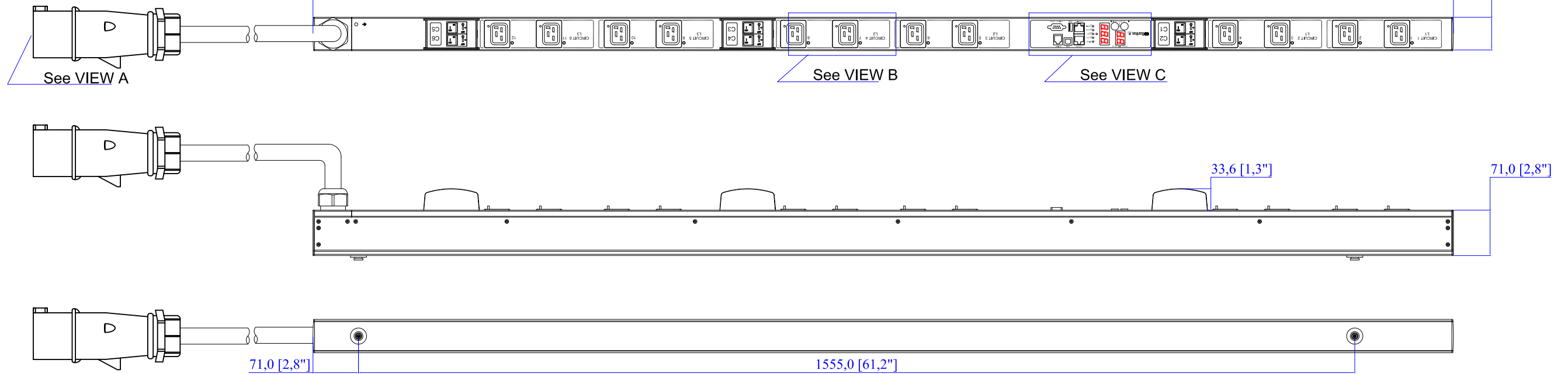
IEC60309 32A 3PY
