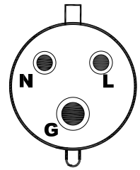
IEC60309 32A PSE
