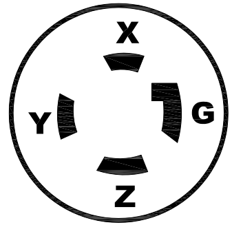
NEMA L15-30P
