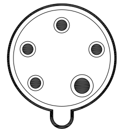
IEC60309 30A 3PY
