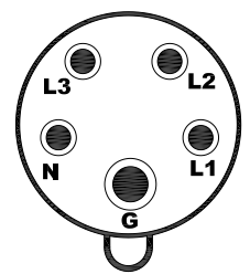
IEC60309 32A 3PY (UL)
