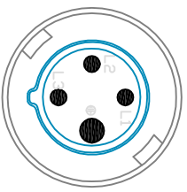
IEC60309 60A
