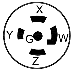
NEMA L21-30P
