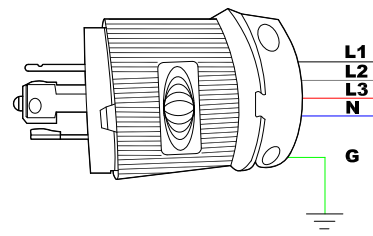
NEMA L22-30P
