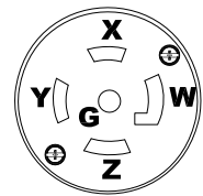
NEMA L22-30P
