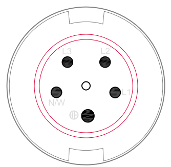
IEC60309 63A
